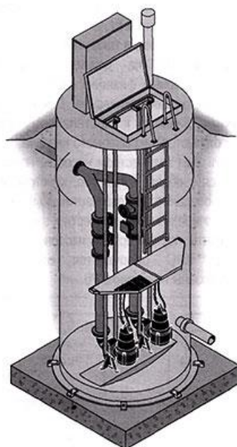
Рис. 7. Комплексы канализационные насосные станции Grundfos
